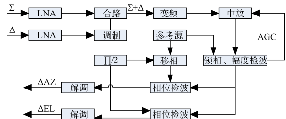
图 1 多模馈源跟踪接收机原理框图
