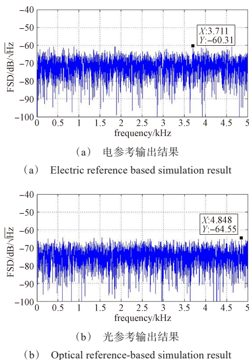
图4 仿真输出的解调噪声功率谱密度图
