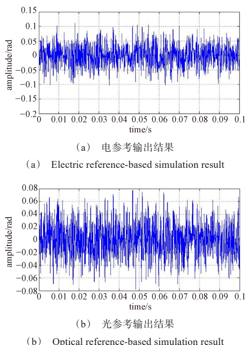
图3 仿真输出的解调噪声时域波形图
