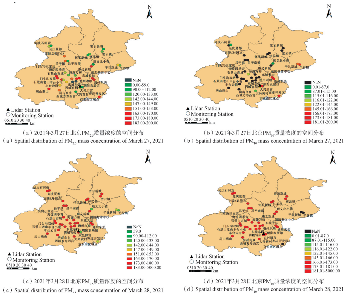
图6 PM_{2.5} 、 PM_{10} 质量浓度空间分布
