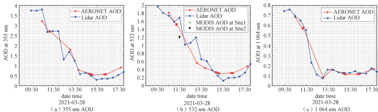
图 7 气溶胶光学厚度比对
