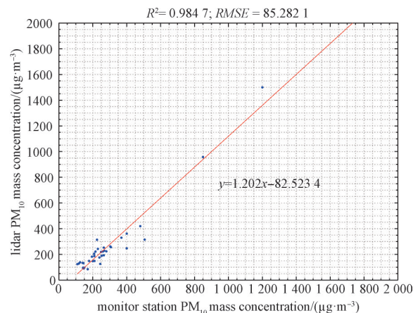
图 10 两观测站点 \text{PM}_{2.5} 、 \text{PM}_{10} 相关性分析
