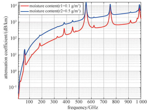
图 3 云雾天气下的信号衰减
