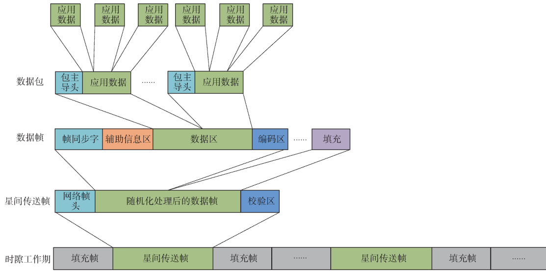
图 9 数据帧结构示意图
