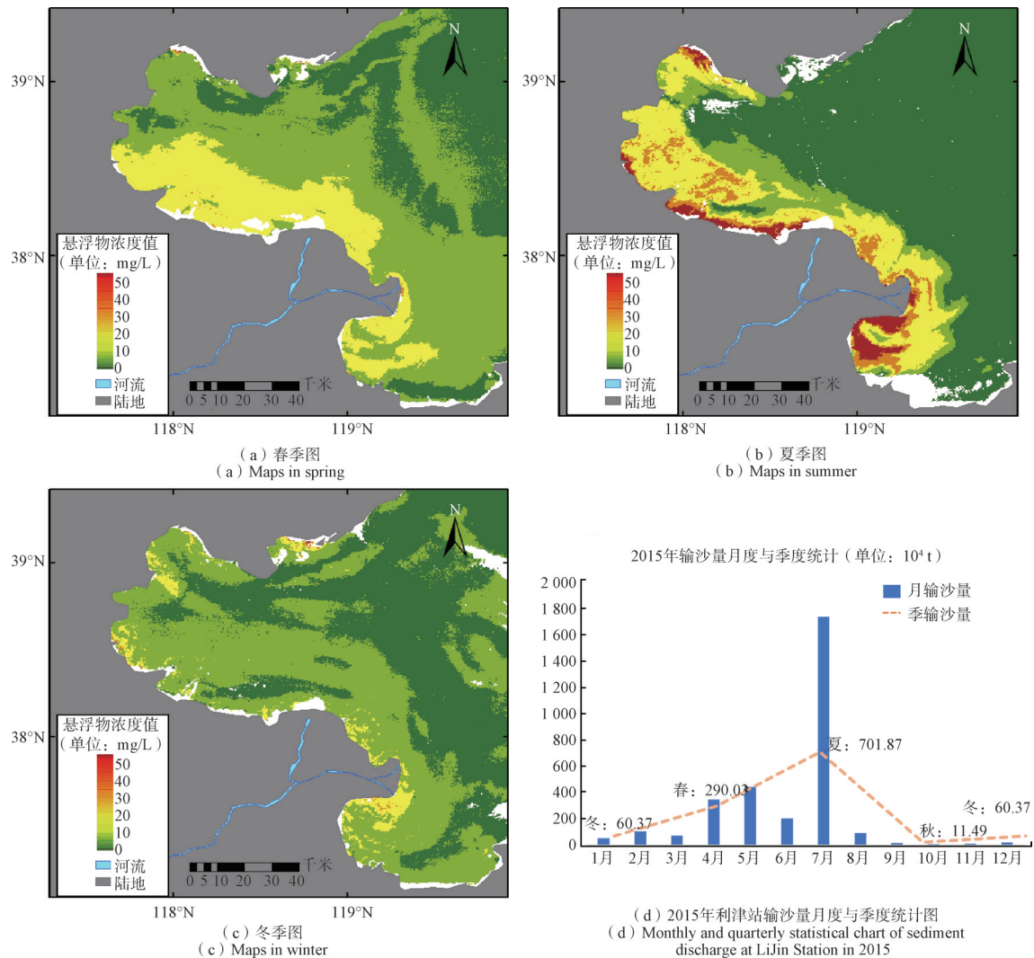
图5 黄河口沿岸海域2015年春季、夏季、冬季悬浮物浓度反演图;2015年利津站输沙量月度与季度统计图
