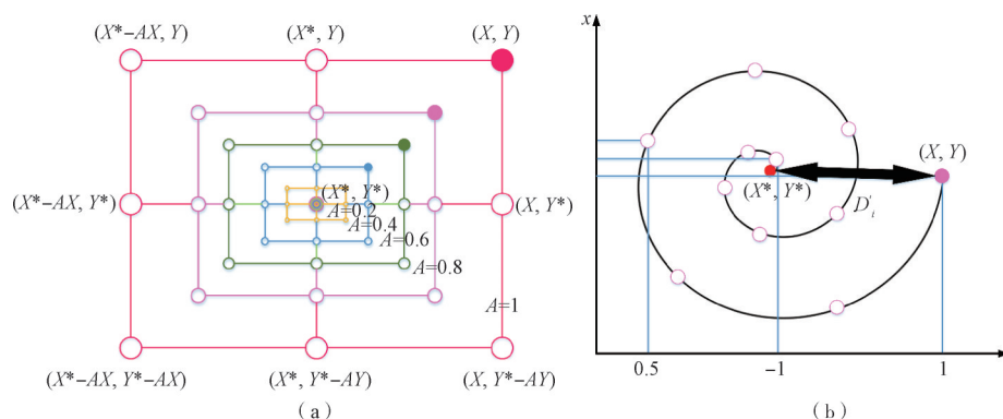
图4 WOA中实现的气泡搜索机制( X^* 为最佳解)
