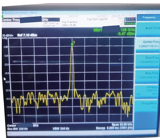
图 10 发射机单载波信号
