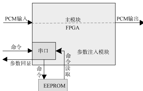
图 5 FPGA 分区工作原理框图
